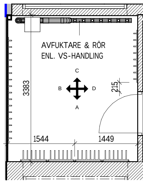
PLAN TORKRUM 1002 1 : 50
